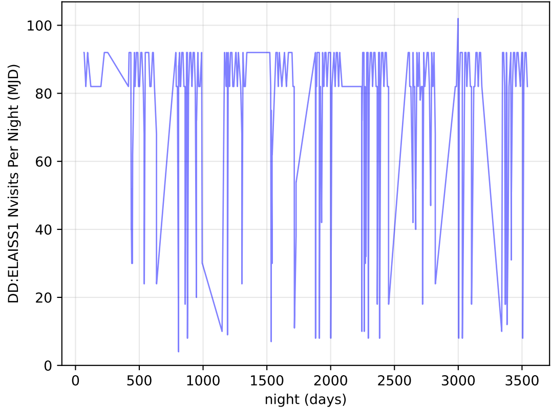
too_elab_r8_d3_ugrizy_v3.4_10yrs all bands: DD:ELAISS1 Nvisits Per Night
