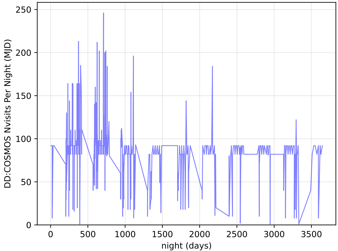
too_elab_r8_d3_ugrizy_v3.4_10yrs all bands: DD:COSMOS Nvisits Per Night
