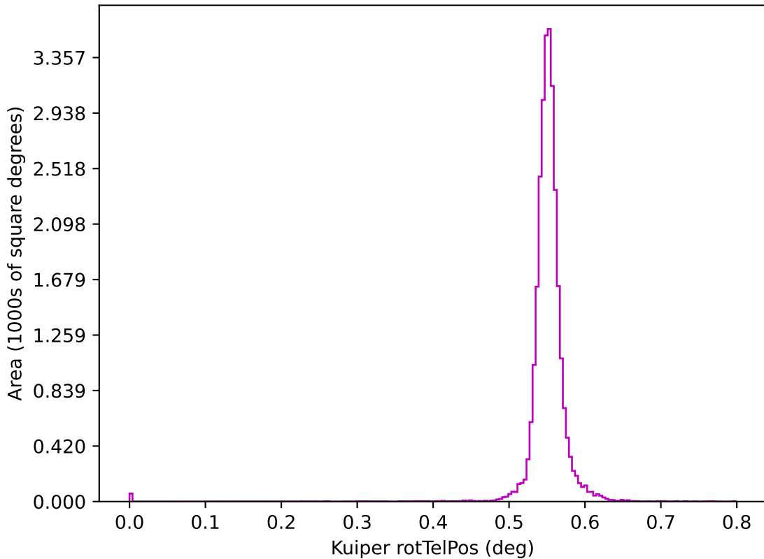
too_elab_r8_d3_gz_v3.4_10yrs z: Kuiper rotTelPos
