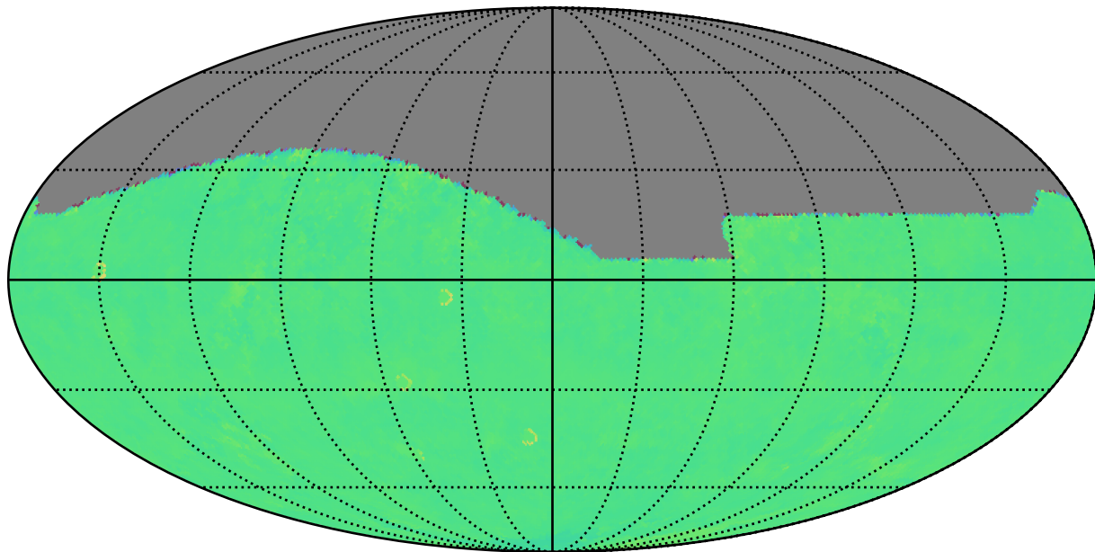
too_elab_r8_d3_gz_v3.4_10yrs i: Kuiper rotTelPos
