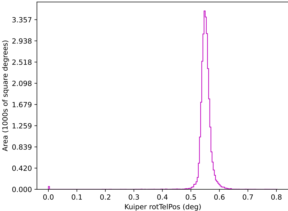
too_elab_r8_d3_griz_v3.4_10yrs z: Kuiper rotTelPos
