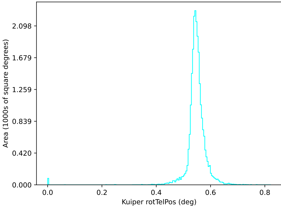
too_elab_r8_d3_griz_v3.4_10yrs u: Kuiper rotTelPos
