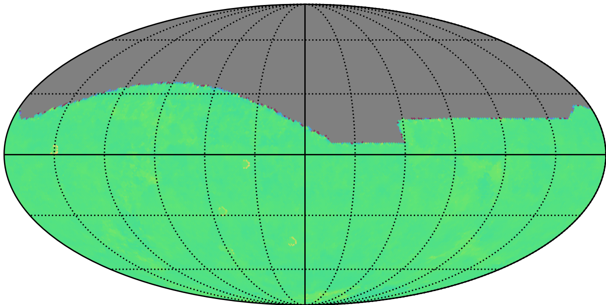
too_elab_r8_d3_griz_v3.4_10yrs i: Kuiper rotTelPos
