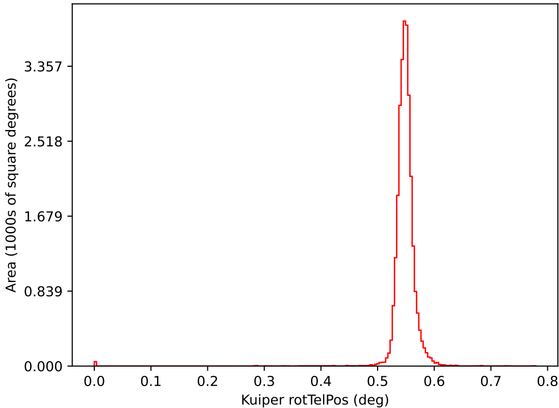
too_elab_r8_d3_griz_v3.4_10yrs i: Kuiper rotTelPos
