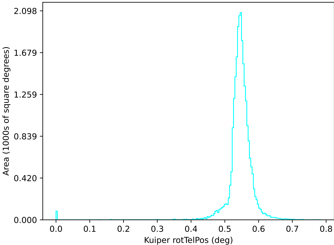
too_elab_r8_d3_giz_v3.4_10yrs u: Kuiper rotTelPos
