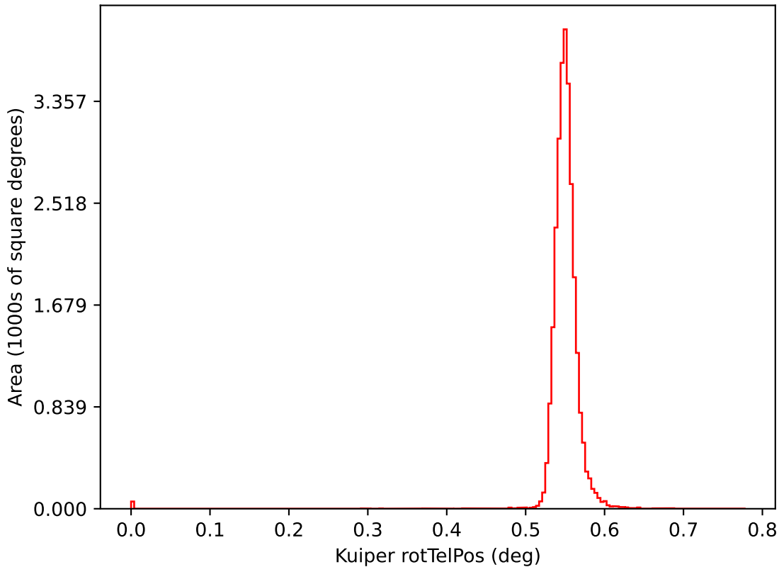
too_elab_r8_d3_giz_v3.4_10yrs i: Kuiper rotTelPos
