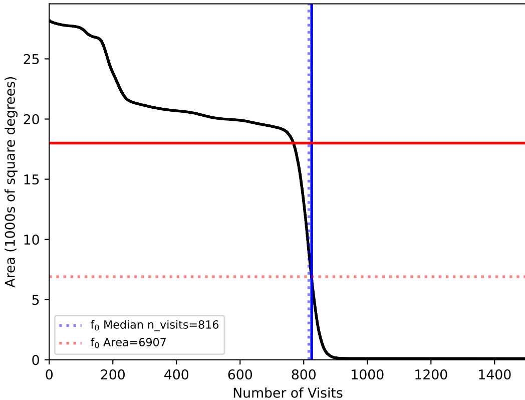
too_elab_r8_d2_ugrizy_v3.4_10yrs : fO
