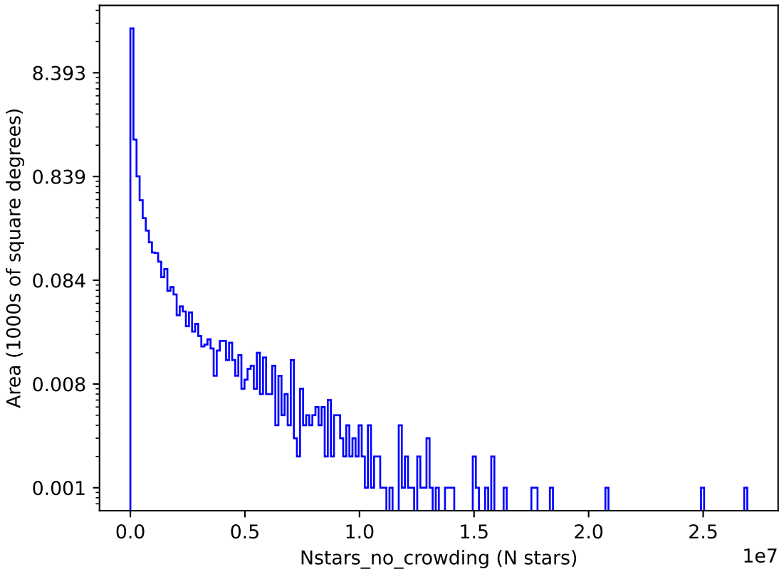
too_elab_r8_d2_ugrizy_v3.4_10yrs i: Nstars_no_crowding
