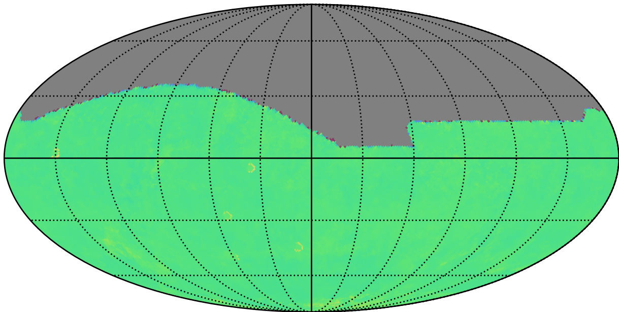
too_elab_r8_d2_ugrizy_v3.4_10yrs r: Kuiper rotTelPos
