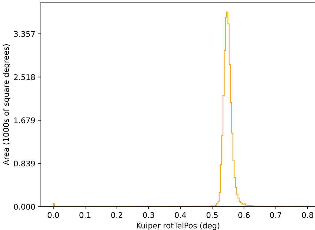
too_elab_r8_d2_ugrizy_v3.4_10yrs r: Kuiper rotTelPos
