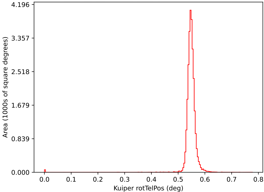
too_elab_r8_d2_ugrizy_v3.4_10yrs i: Kuiper rotTelPos
