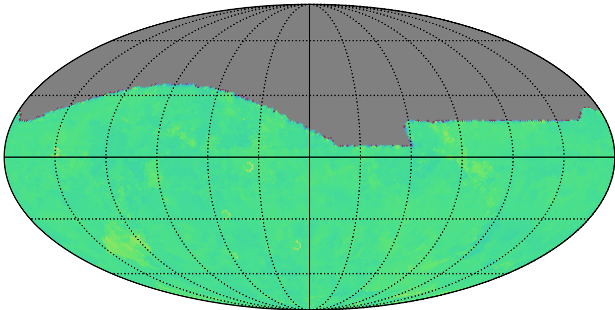
too_elab_r8_d2_ugrizy_v3.4_10yrs g: Kuiper rotTelPos
