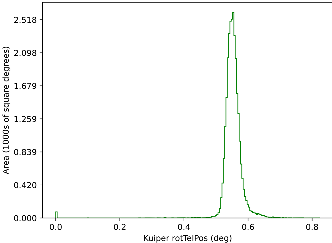
too_elab_r8_d2_ugrizy_v3.4_10yrs g: Kuiper rotTelPos
