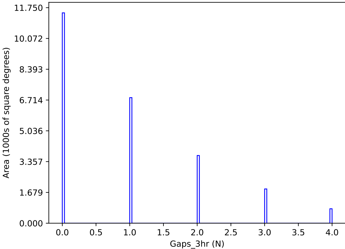
too_elab_r8_d2_ugrizy_v3.4_10yrs y band: Gaps_3hr
