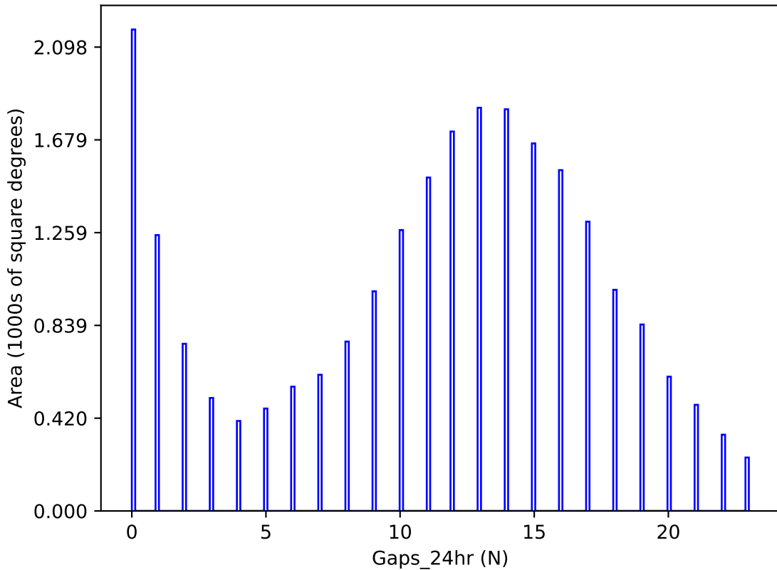
too_elab_r8_d2_ugrizy_v3.4_10yrs y band: Gaps_24hr
