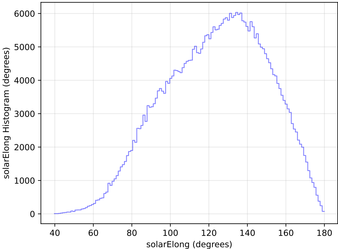
too_elab_r8_d2_ugrizy_v3.4_10yrs WFD y band: solarElong Histogram
