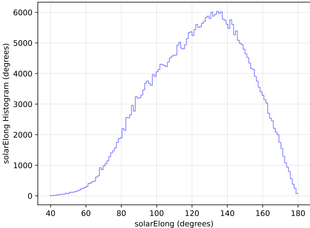
too_elab_r8_d2_ugrizy_v3.4_10yrs All sky y band: solarElong Histogram
