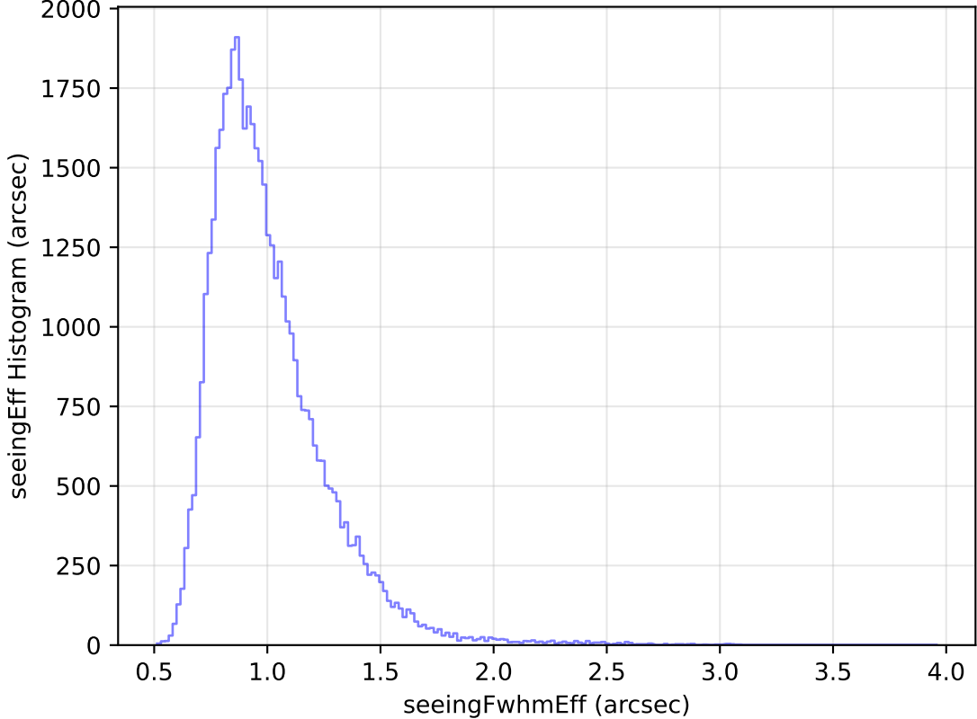
too_elab_r8_d2_ugrizy_v3.4_10yrs Yr 1 y band: seeingEff Histogram
