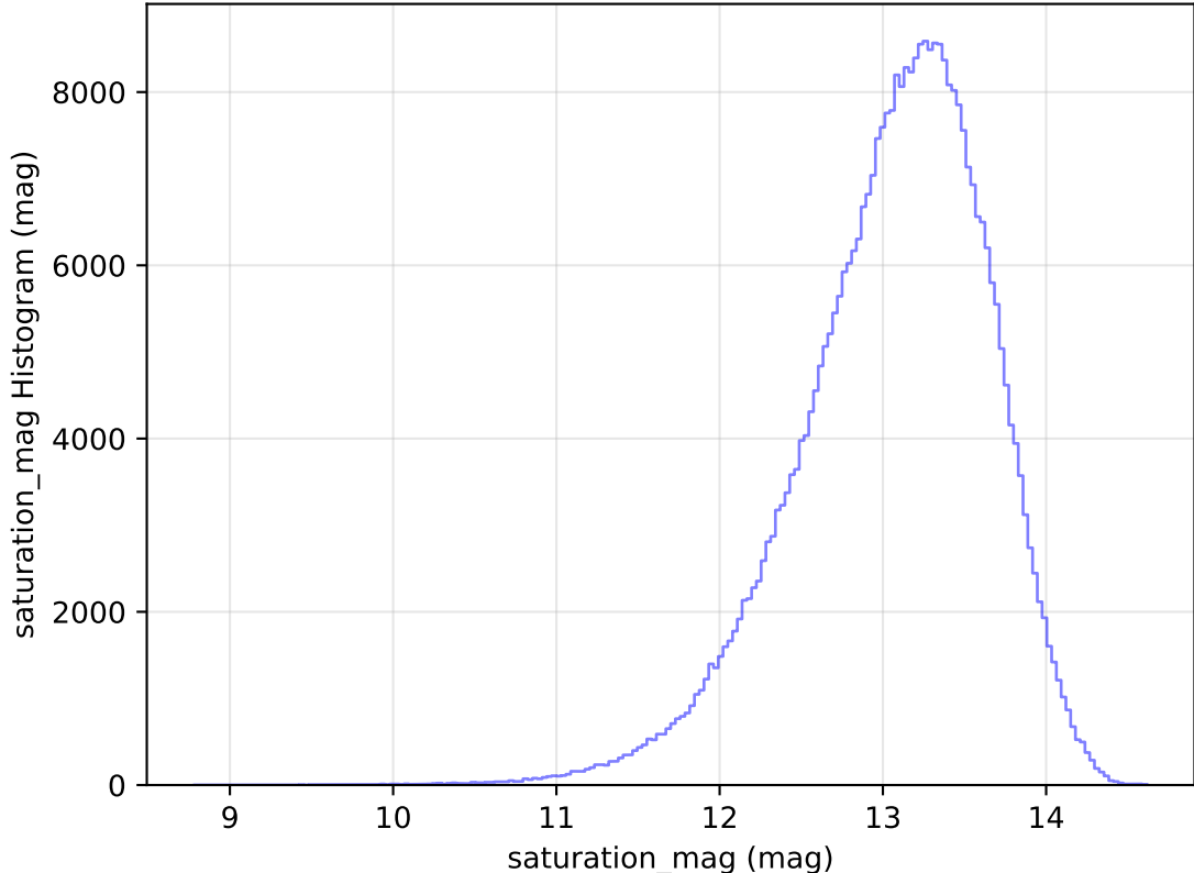
too_elab_r8_d2_ugrizy_v3.4_10yrs All sky y band: saturation_mag Histogram
