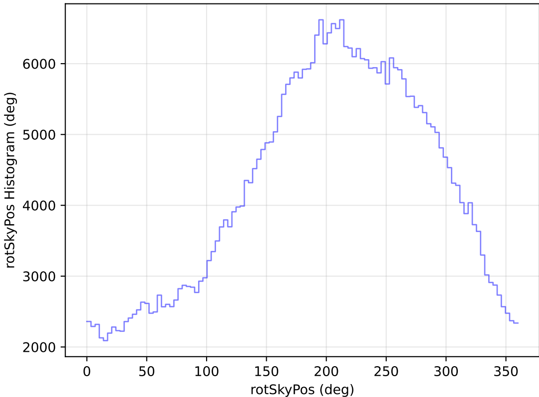
too_elab_r8_d2_ugrizy_v3.4_10yrs WFD z band: rotSkyPos Histogram
