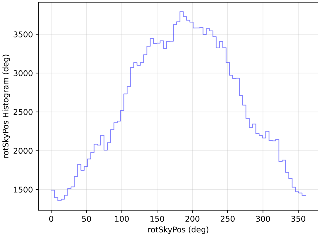
too_elab_r8_d2_ugrizy_v3.4_10yrs WFD g band: rotSkyPos Histogram
