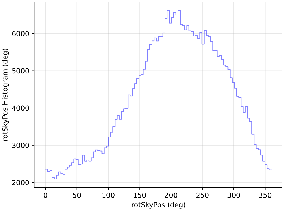
too_elab_r8_d2_ugrizy_v3.4_10yrs All sky z band: rotSkyPos Histogram
