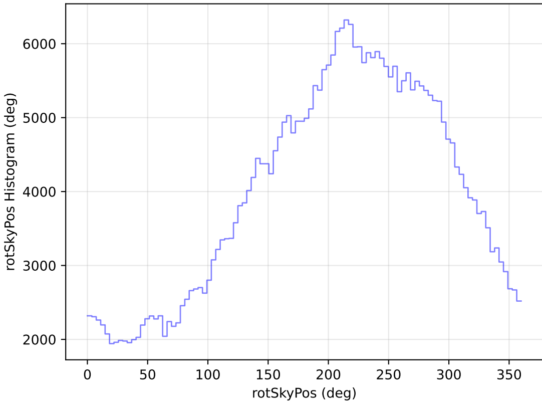
too_elab_r8_d2_ugrizy_v3.4_10yrs All sky y band: rotSkyPos Histogram
