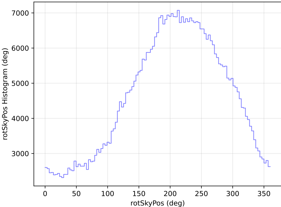
too_elab_r8_d2_ugrizy_v3.4_10yrs All sky i band: rotSkyPos Histogram
