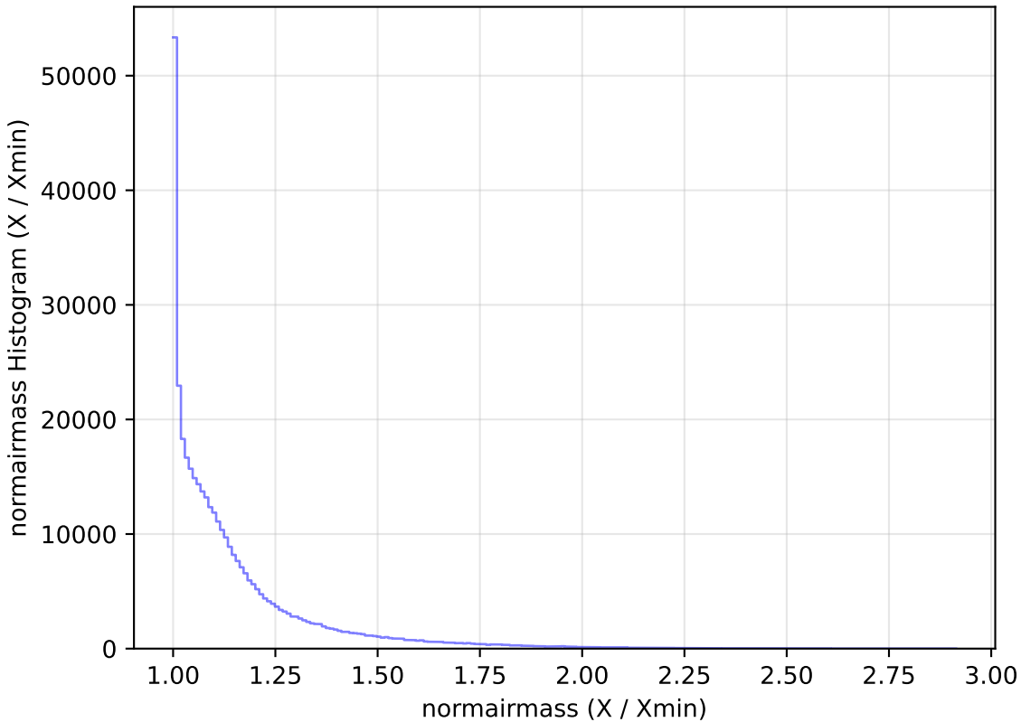
too_elab_r8_d2_ugrizy_v3.4_10yrs WFD y band: normairmass Histogram
