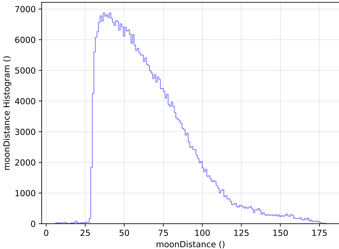
too_elab_r8_d2_ugrizy_v3.4_10yrs WFD y band: moonDistance Histogram
