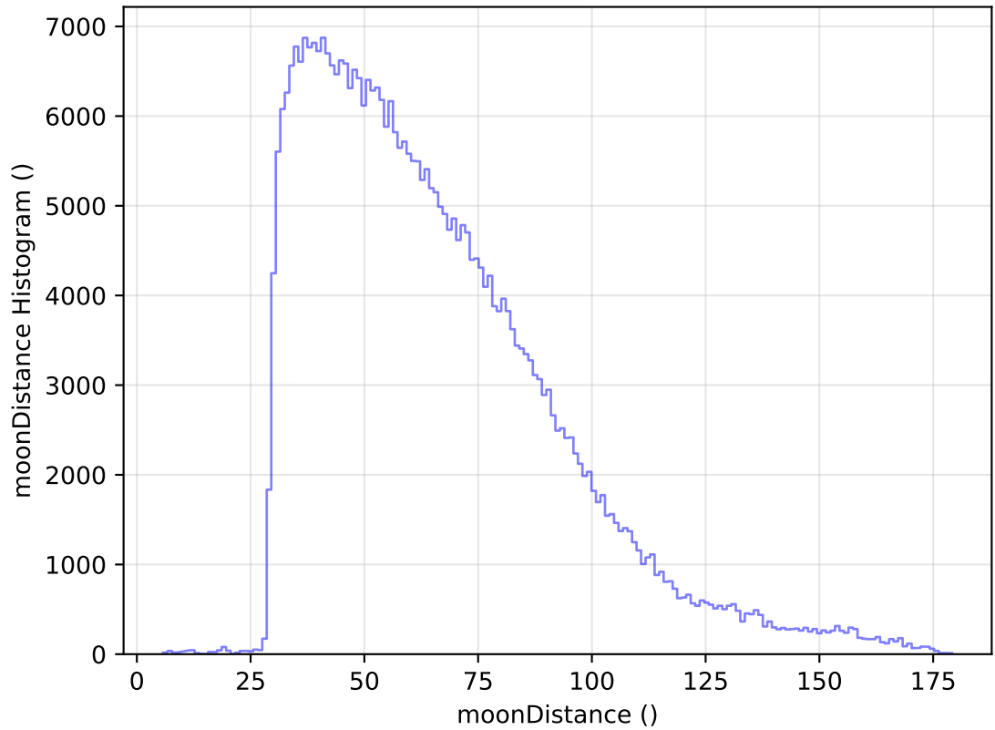
too_elab_r8_d2_ugrizy_v3.4_10yrs All sky y band: moonDistance Histogram
