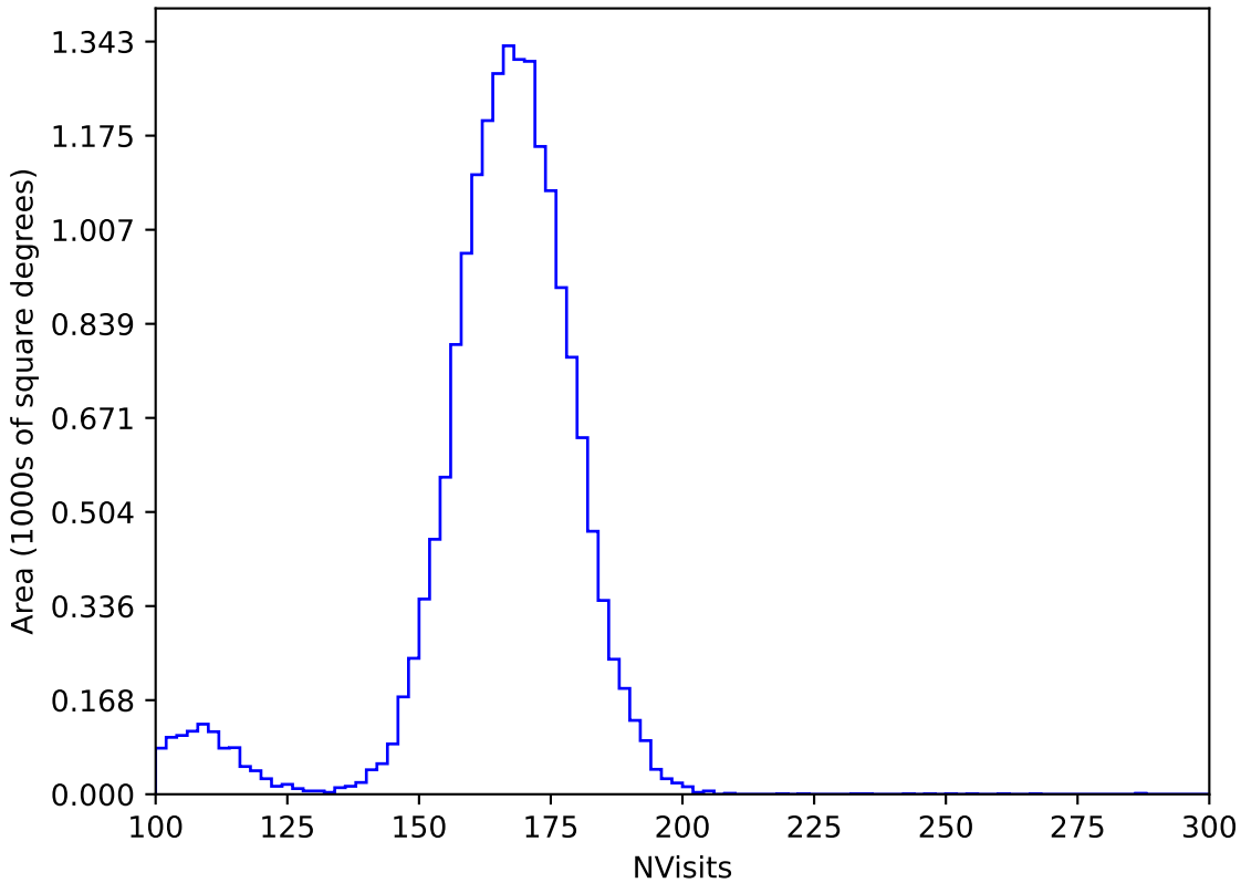
too_elab_r8_d2_ugrizy_v3.4_10yrs WFD y band: NVisits
