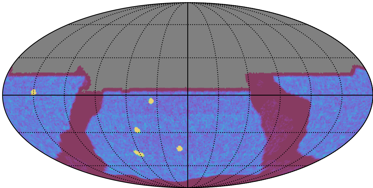
too_elab_r8_d2_ugrizy_v3.4_10yrs All sky y band: NVisits
