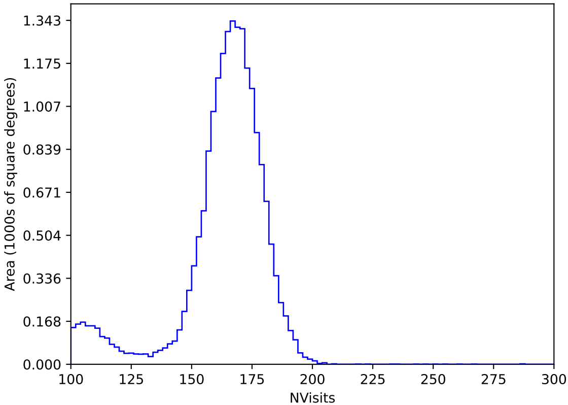
too_elab_r8_d2_ugrizy_v3.4_10yrs All sky y band: NVisits
