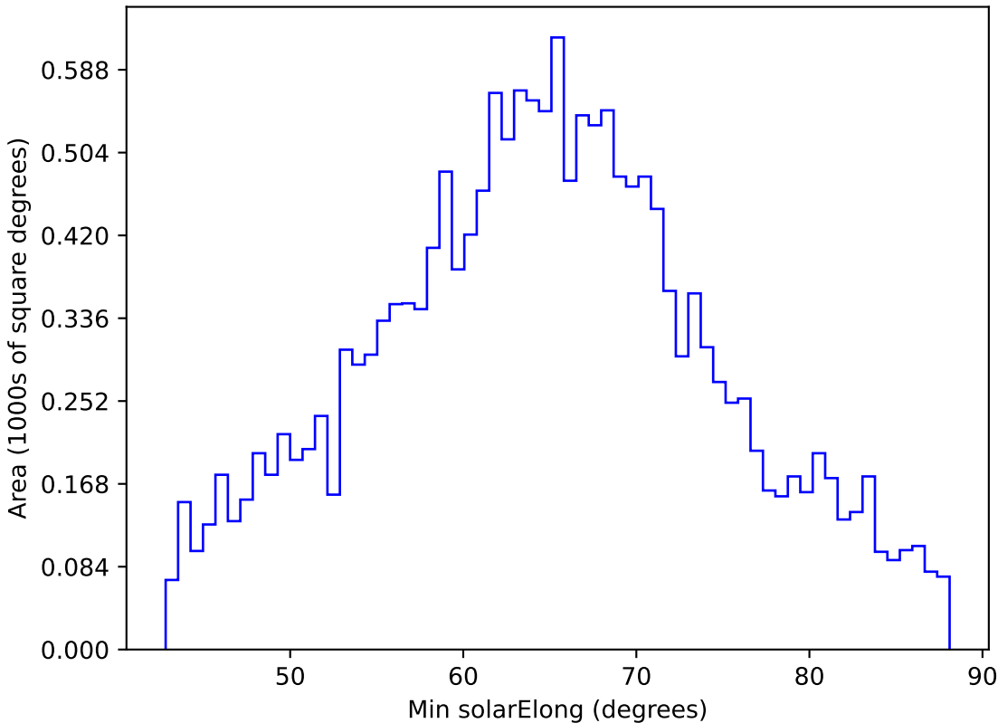
too_elab_r8_d2_ugrizy_v3.4_10yrs WFD y band: Min solarElong
