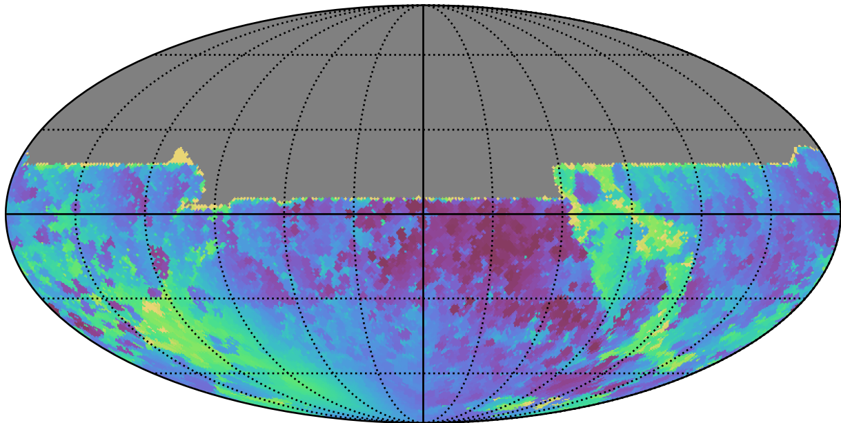
too_elab_r8_d2_ugrizy_v3.4_10yrs All sky y band: Min solarElong
