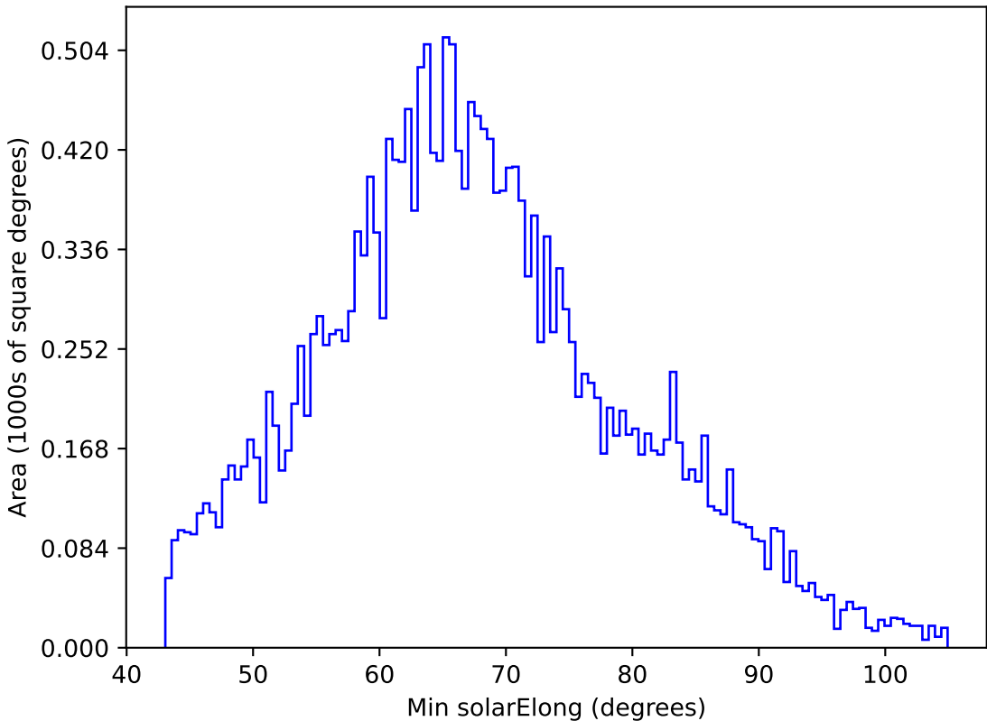
too_elab_r8_d2_ugrizy_v3.4_10yrs All sky y band: Min solarElong
