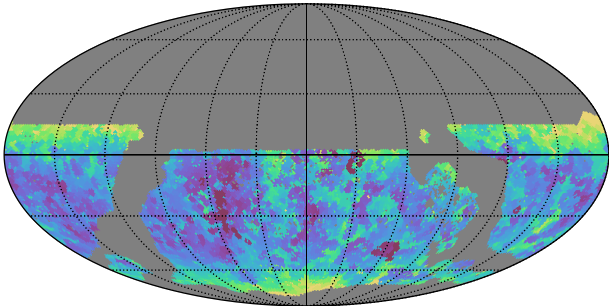
too_elab_r8_d2_ugrizy_v3.4_10yrs WFD y band: Min seeingEff
