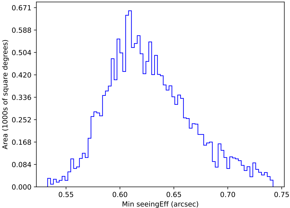
too_elab_r8_d2_ugrizy_v3.4_10yrs WFD y band: Min seeingEff
