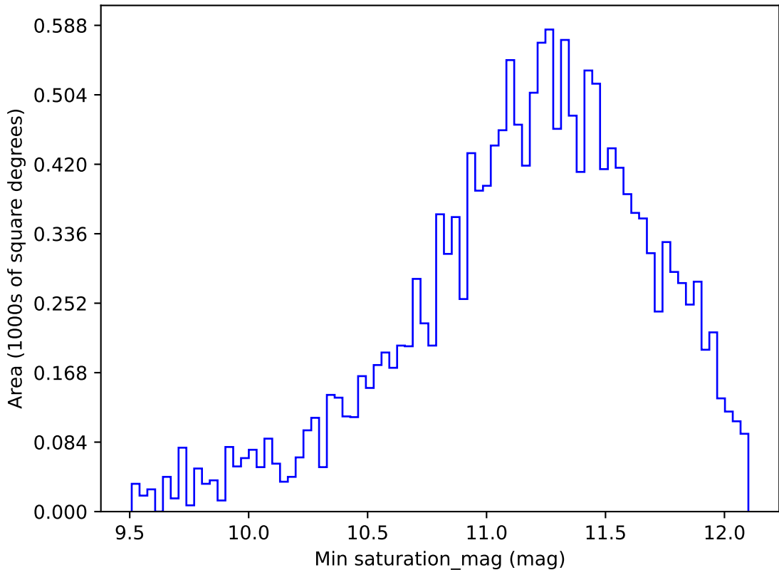
too_elab_r8_d2_ugrizy_v3.4_10yrs WFD y band: Min saturation_mag
