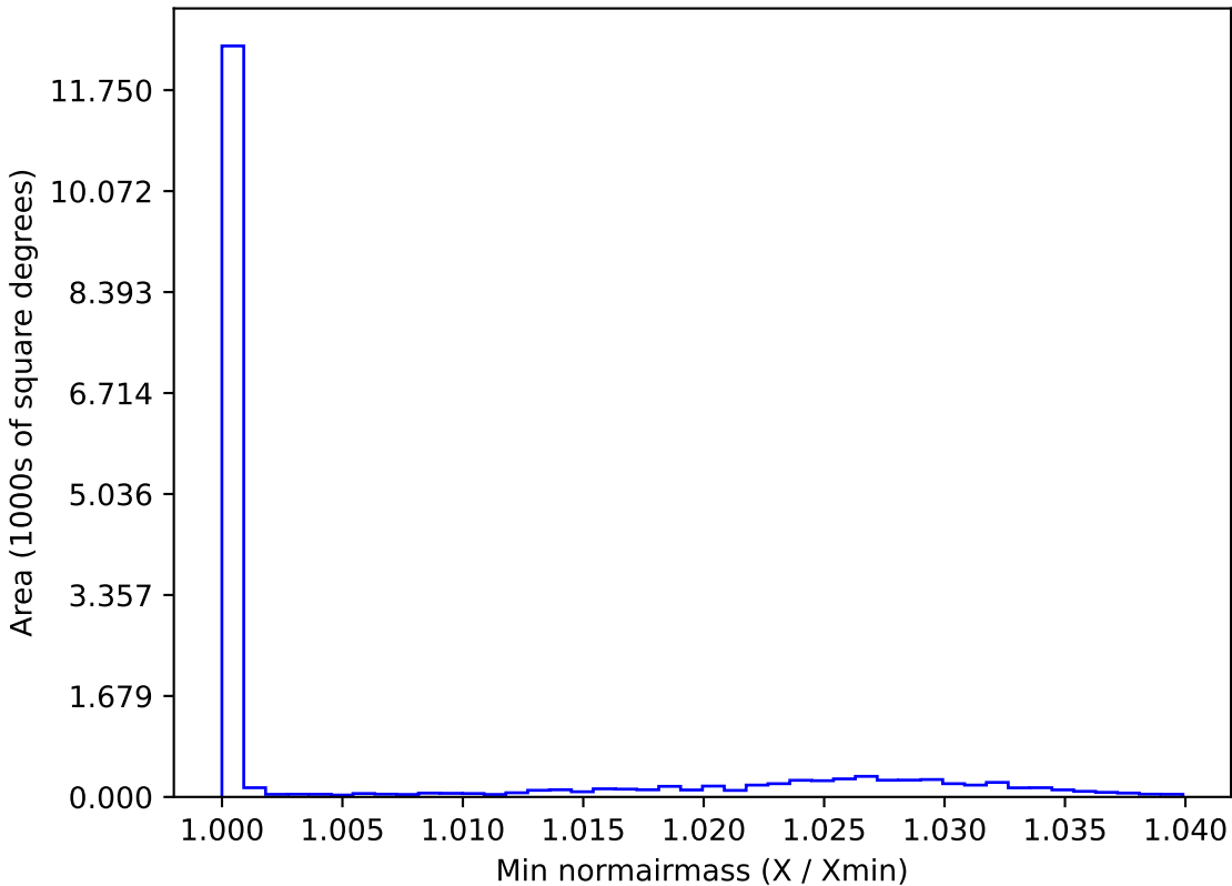
too_elab_r8_d2_ugrizy_v3.4_10yrs WFD y band: Min normairmass
