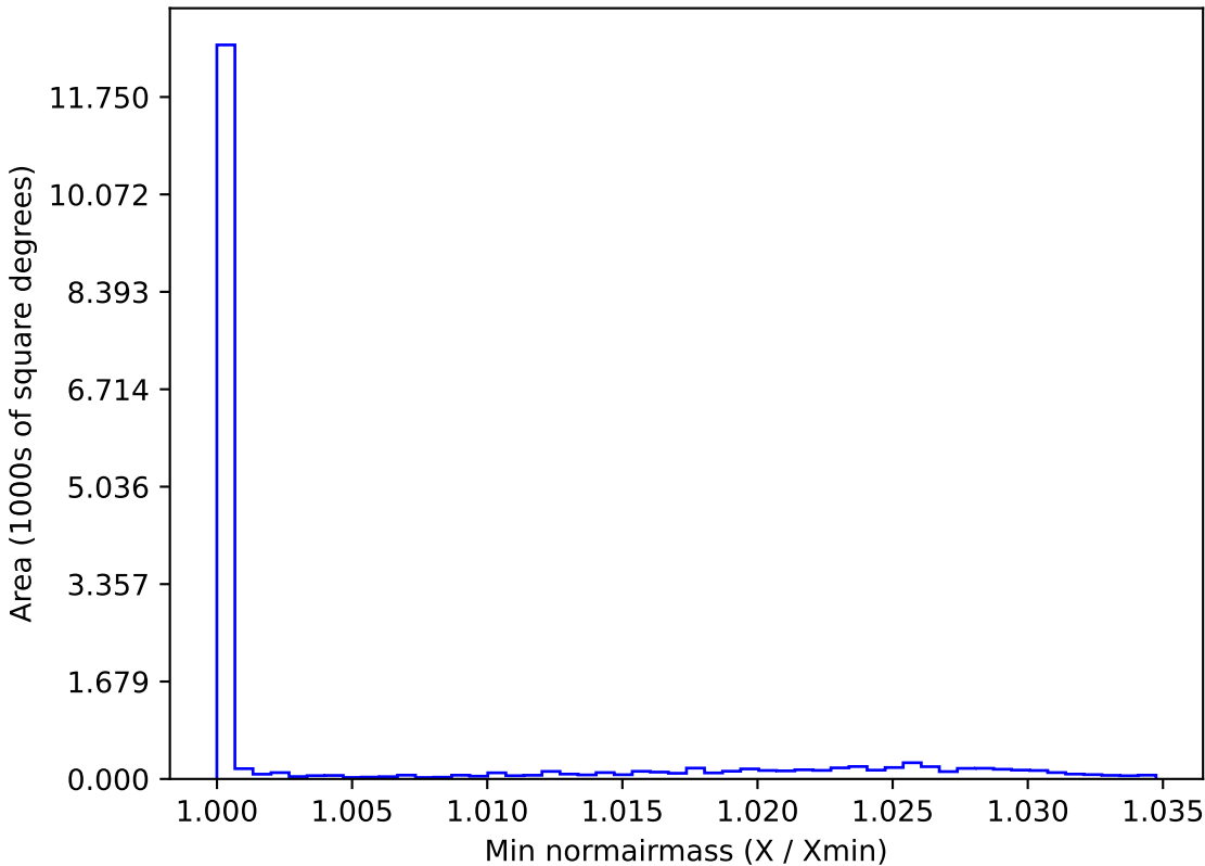
too_elab_r8_d2_ugrizy_v3.4_10yrs WFD i band: Min normairmass
