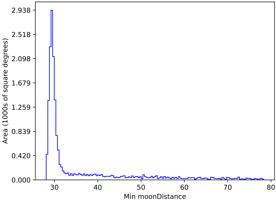
too_elab_r8_d2_ugrizy_v3.4_10yrs WFD y band: Min moonDistance
