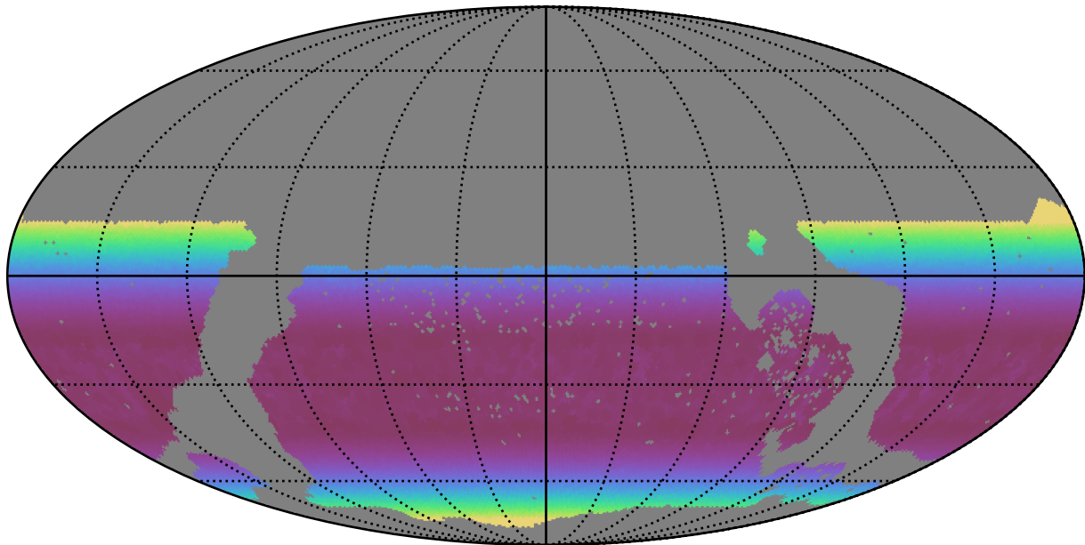
too_elab_r8_d2_ugrizy_v3.4_10yrs WFD y band: Min airmass
