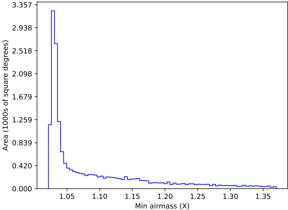
too_elab_r8_d2_ugrizy_v3.4_10yrs WFD y band: Min airmass
