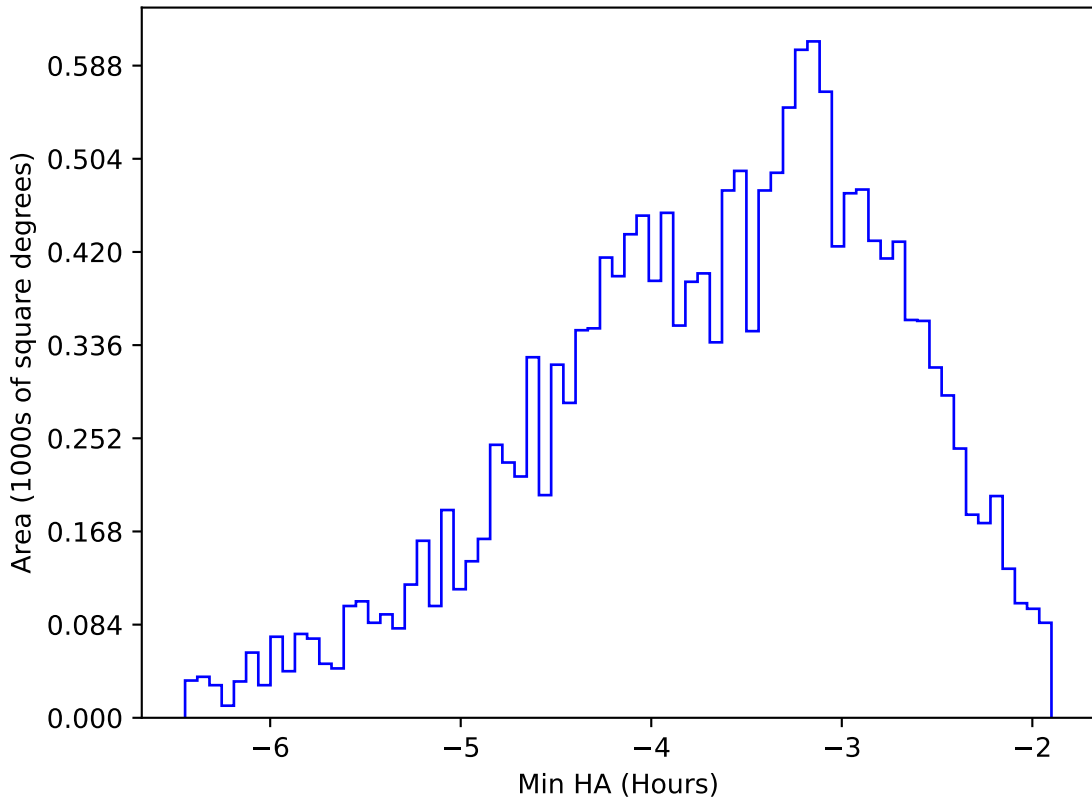
too_elab_r8_d2_ugrizy_v3.4_10yrs WFD y band: Min HA
