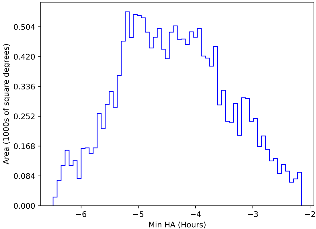
too_elab_r8_d2_ugrizy_v3.4_10yrs WFD i band: Min HA
