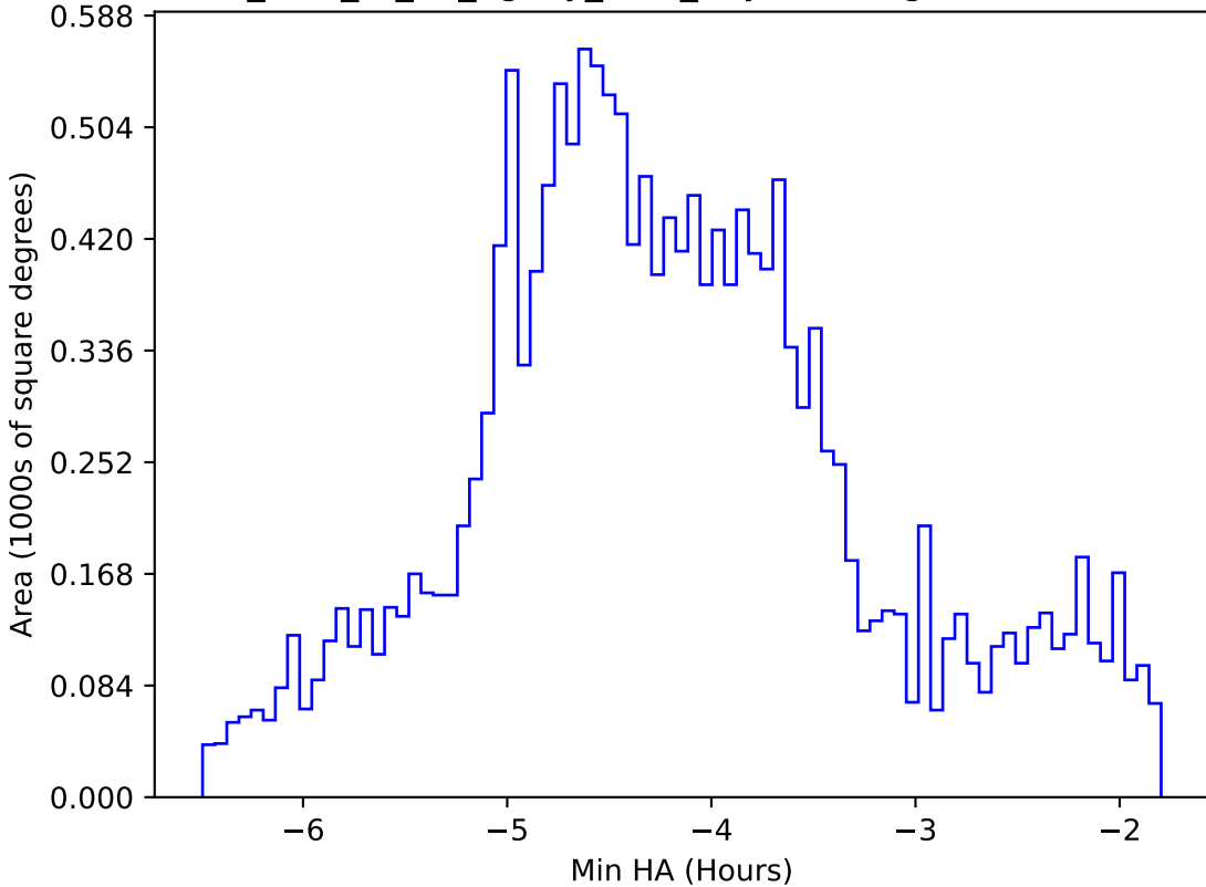
too_elab_r8_d2_ugrizy_v3.4_10yrs WFD g band: Min HA
