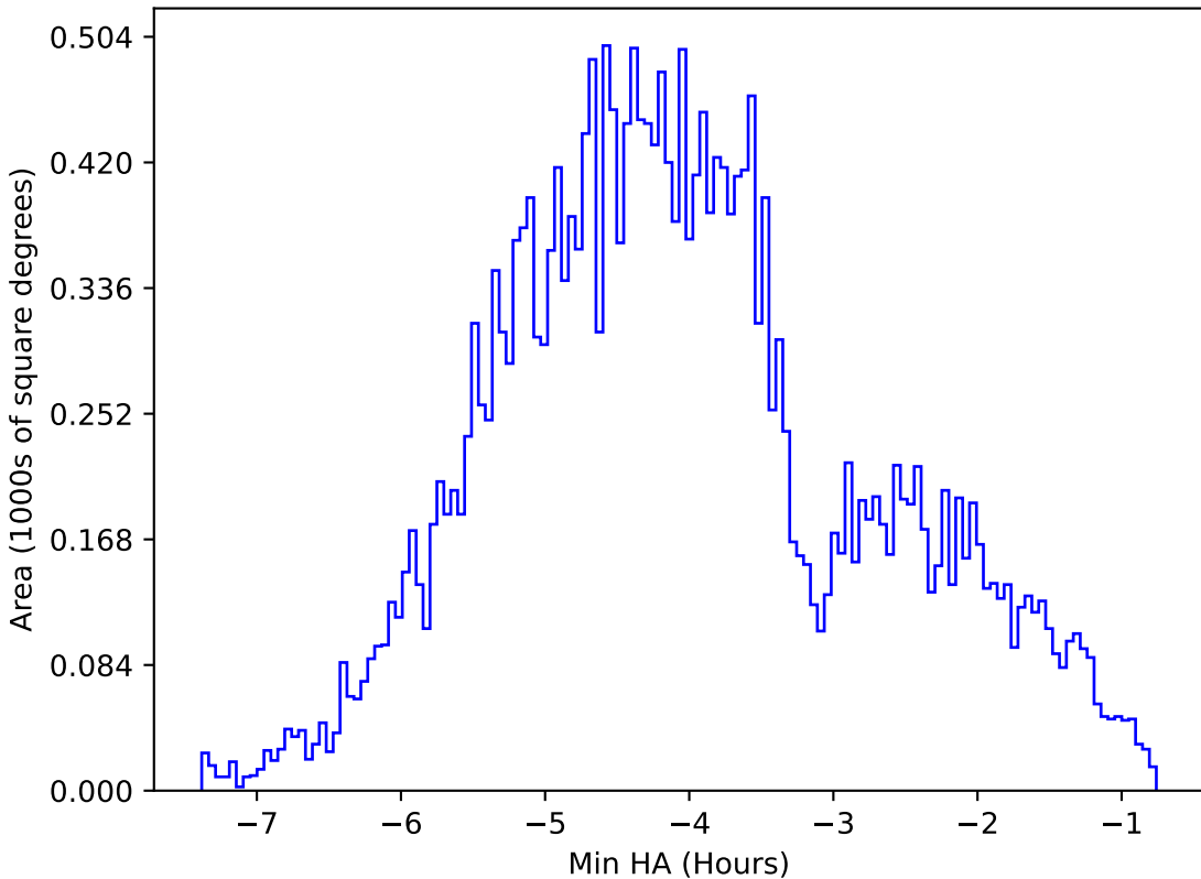
too_elab_r8_d2_ugrizy_v3.4_10yrs All sky z band: Min HA
