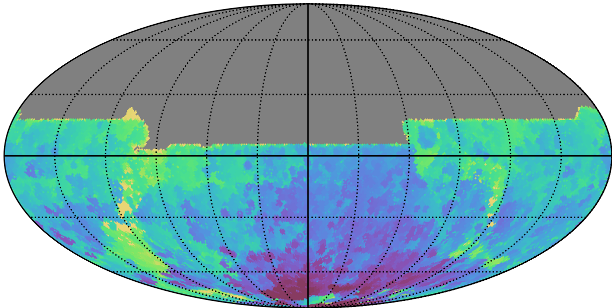
too_elab_r8_d2_ugrizy_v3.4_10yrs All sky y band: Min HA
